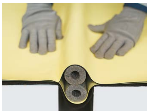
Рис. 6. Монтаж гидроизоляционной мембраны в месте расположения деформационных швов
