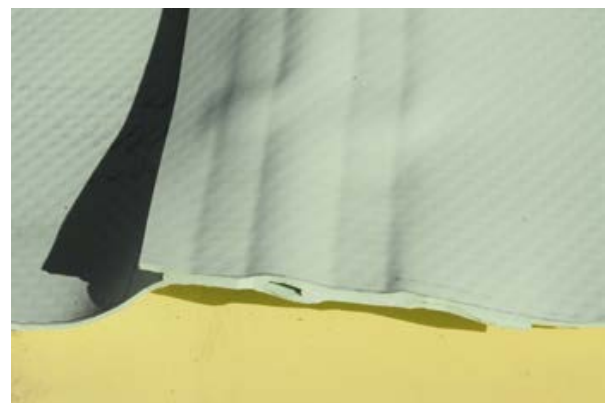
Рис. 11. Сварка полотен текстурированной мембраны (2-го слоя) при помощи автоматического оборудования, позволяющего создать двойной шов с проверочным каналом
