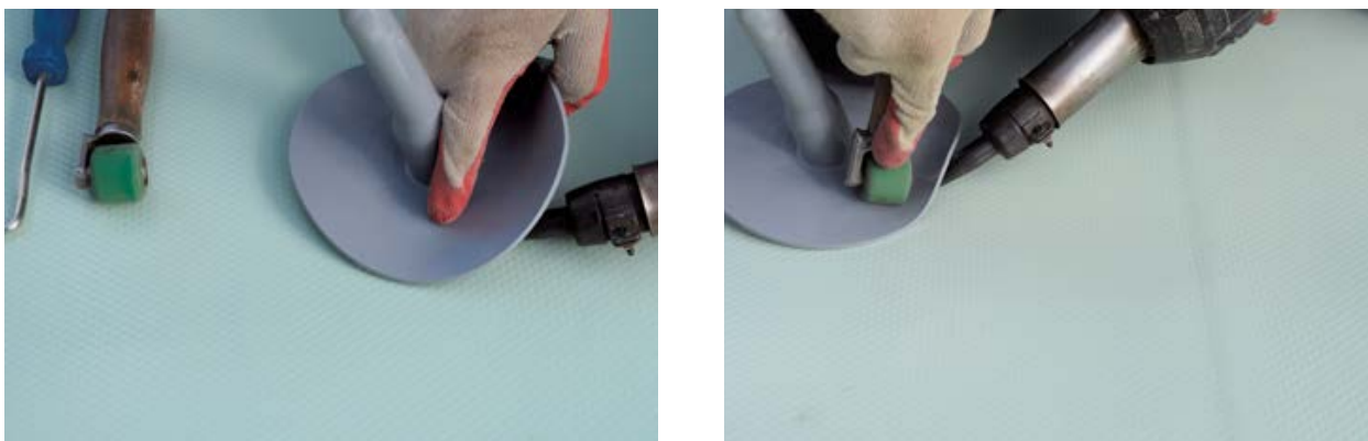
Рис. 18. Монтаж ПВХ инъекционного штуцера с помощью ручного сварочного аппарата
