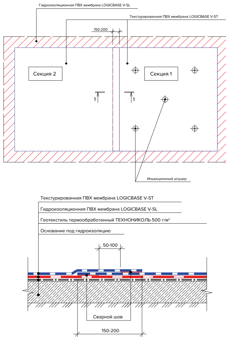
Рис. 16. Устройство перехлестов текстурированной мембраны между секциями на схемах и узлах чертежей
