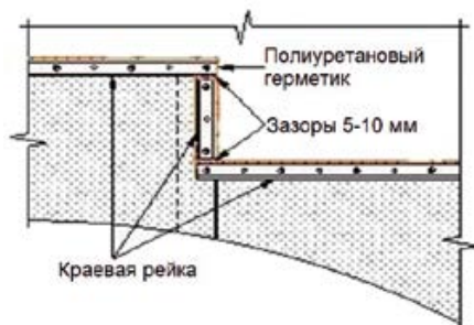
Рис. 26. Обрамление края кровельного ковра краевой рейкой
