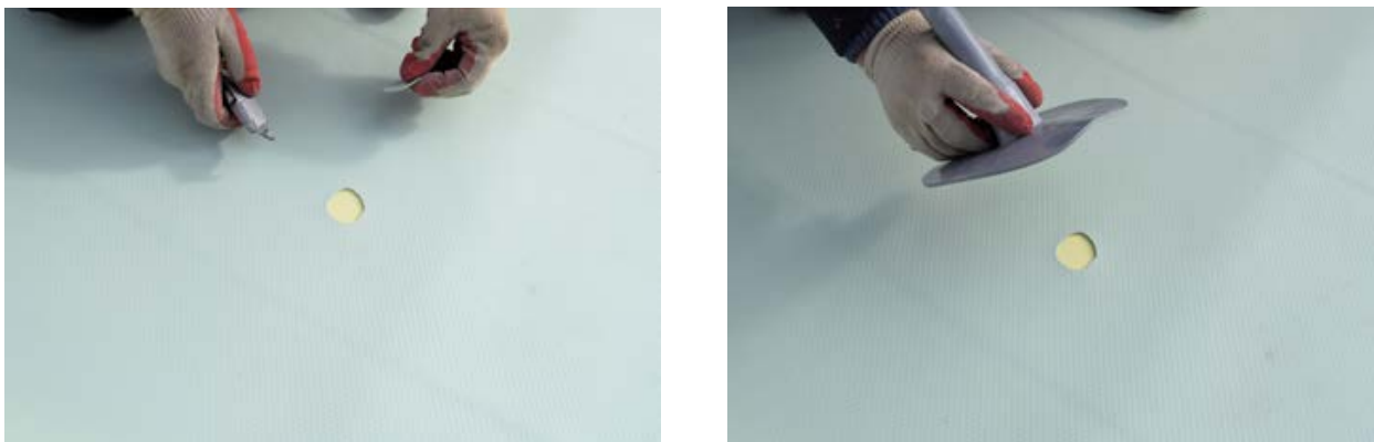
Рис. 17. Пример подготовки отверстия под монтаж ПВХ инъекционного штуцера с помощью ножа-крючка
