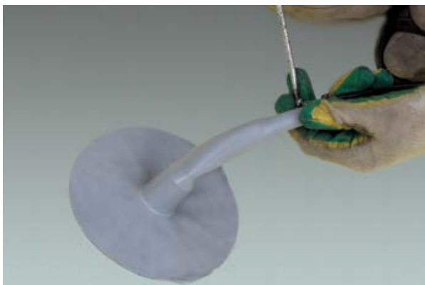
Рис. 20. Соединение прямого инъекционного штуцера и трубки
