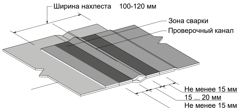
Рис. 7. Двойной шов с проверочным каналом
